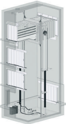
Ohne Maschinenraum (MRL) Antrieb in der Schachtgrube
